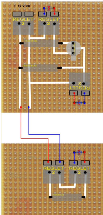
Delante, lado componentes
