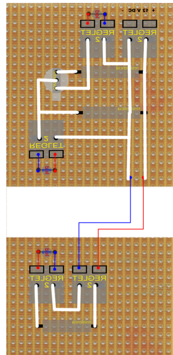
Detrás, lado soldaduras
